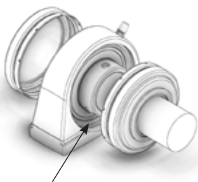
Scanalatura di montaggio lavorata e non verniciata
