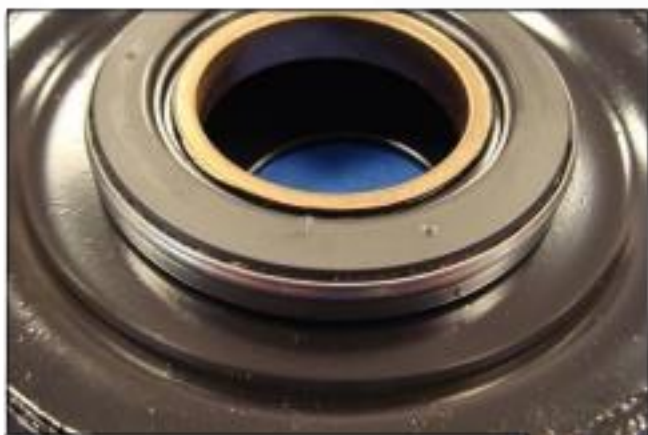
Richtiger Einbau des Federbeinlagers
