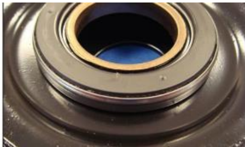
Montaje correcto del axial
