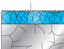
Abb. 11: Schnittansicht der phosphatierten Schicht des Stahlblechkäfigs
