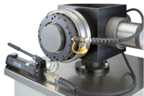
Montage auf Spannhülse mit einer Hydraulikmutter
