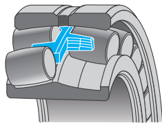
Abb. 12: Ultage-Ausführung mit Messingmassivkäfig
