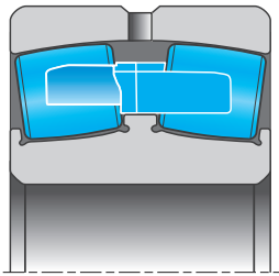
Abb. 7: Querschnitt eines Wälzlagers Typ B
