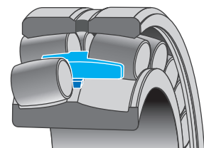
Abb. 6: ULTAGE-Ausführung für große Wälzlager
