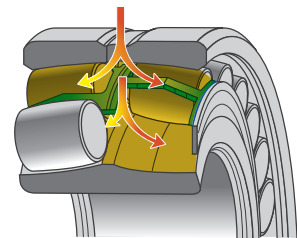
Abb. 5: Besserer Schmiermittelfluss im Wälzlager
