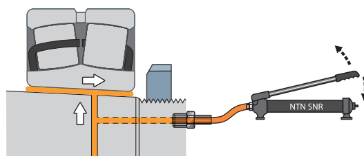
Prinzip der hydraulischen Demontage bei vorhandenen Hydraulikbohrungen und -nuten
