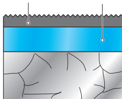
Abb. 10: Schnittansicht der nitrierten Schicht des Stahlblechkäfigs
