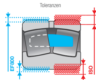
Abb. 16: Spezielle Toleranzen für Außendurchmesser und Bohrung
