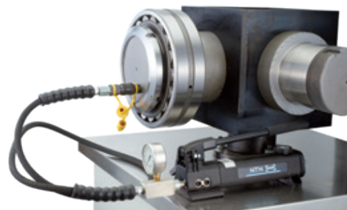
Hydraulische Demontage
