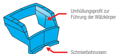
Abb. 15: Perfekte Führung der Wälzkörper durch elastisches Material mit niedrigem Reibungskoeffizienten
