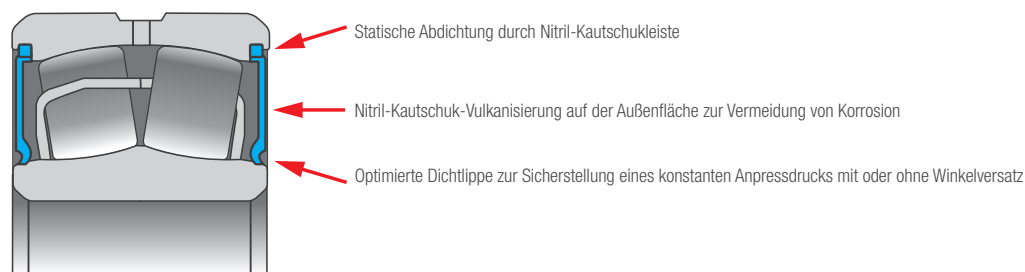
Abb. 17: ULTAGE-Pendelrollenlager mit EE-Dichtung
