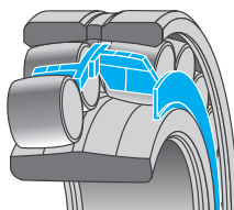
Abb. 14: Ausführung Ultage mit Polyamidkäfig
