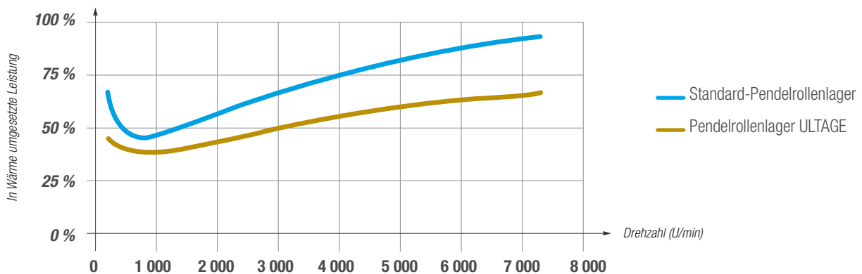
Abb. 2: Gegenüberstellung von in Wärme umgesetzter Leistung und der Drehzahl.
