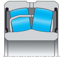
Abb. 4: Querschnitt der Ultage-Konstruktion mit Käfig aus tiefgezogenem Stahl (EA)
