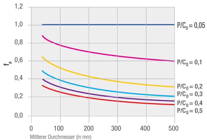
Diagramm 2: Berichtigungsfaktor f_p
