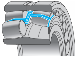
Abb. 8: Ultage-Lager mit Stahlblechkäfig
