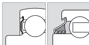
Уплътнение А
